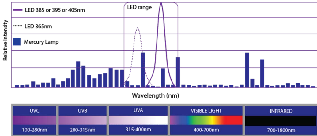
图 6 UV LED 光源与汞灯比较：UV LED = 窄幅高功率 UVA 输出
