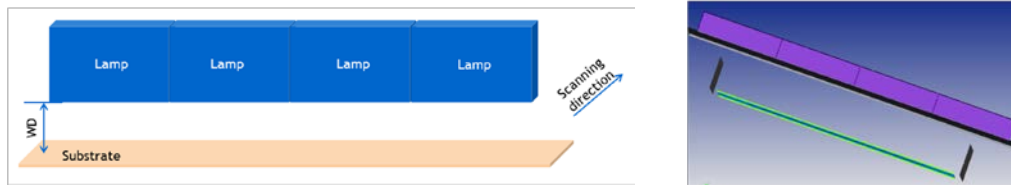
图 8 扫描固化系统设计
