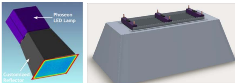
图 7 区域固化 LED 系统设计
