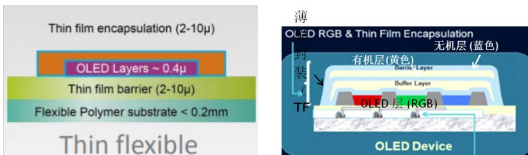
图 2 用于柔性 OLED 的薄膜封装
