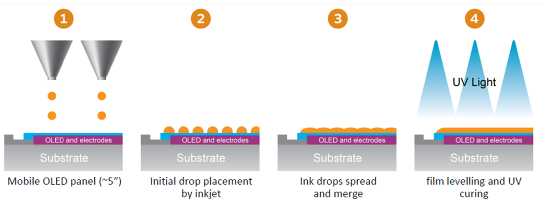
图 4 喷墨印刷薄膜封装 (TFE) 工艺中液体有机层的固化
