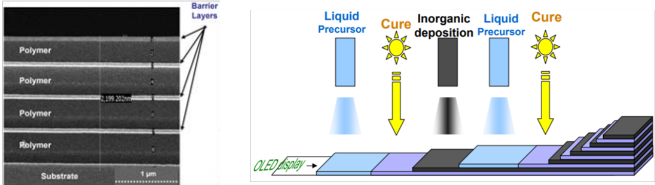
图 3 在 Vitex 工艺中对无机沉积进行固化
