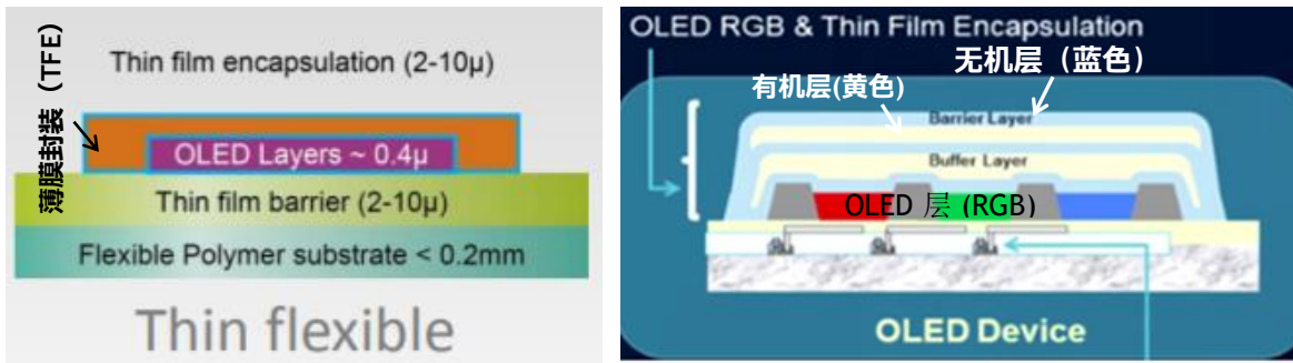
图 2: 用于柔性 OLED 的薄膜封装
