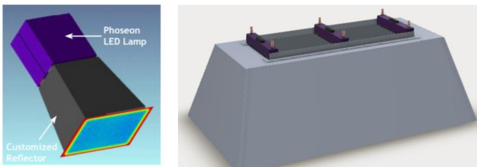
图 7: 区域固化 LED 系统设计
