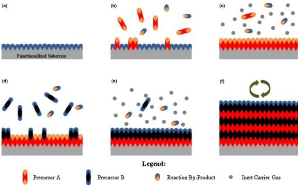
图 5: 原子层沉积法 (ALD) 薄膜封装 (TFE) 工艺
