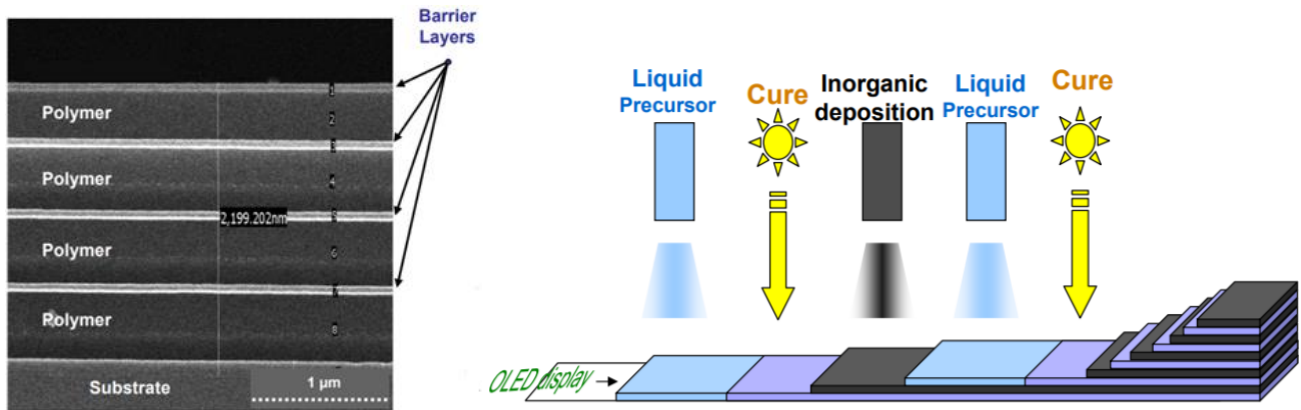
图 3: 在 Vitex 工艺中对无机沉积进行固化
