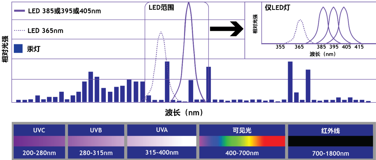
图 6: Output UV LED 与汞的比较 : UV LED =窄幅高功率 UVA 输出
