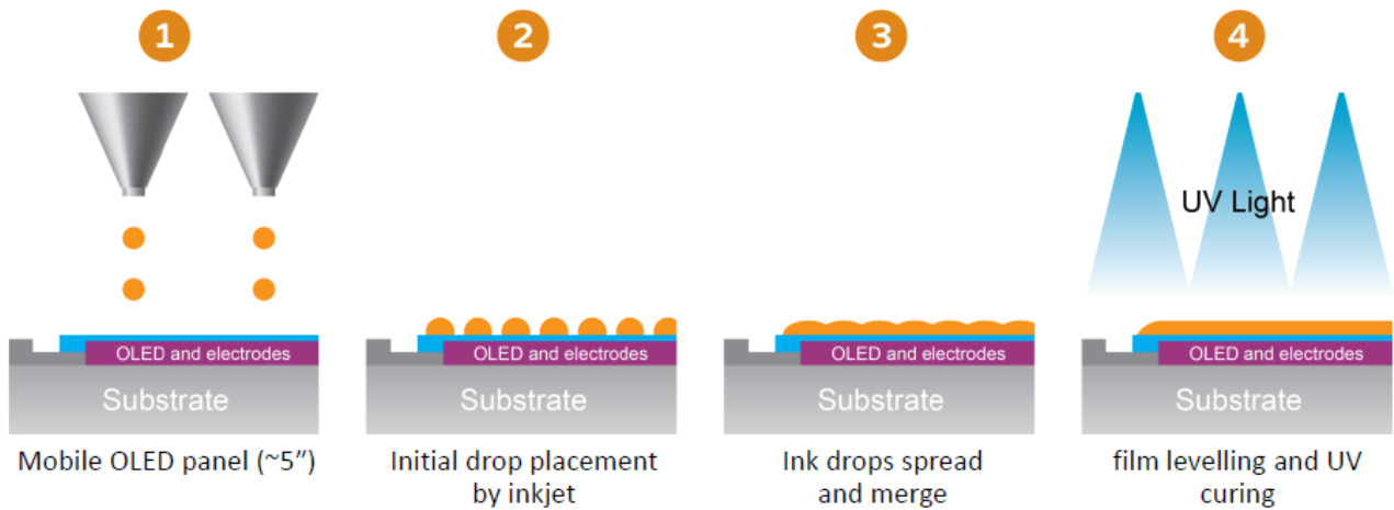
图 4: 喷墨印刷薄膜封装 (TFE) 工艺中液体有机层的固化
